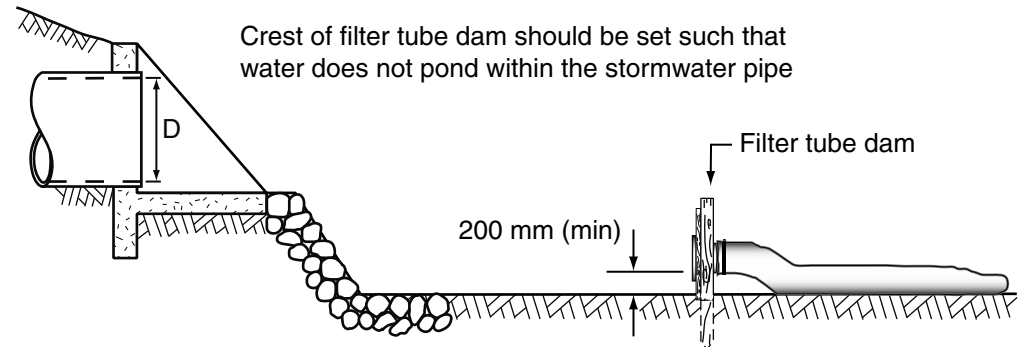
(d) Filter tube dam outlet sediment trap
