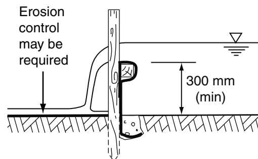
(d) Spill-through weir
